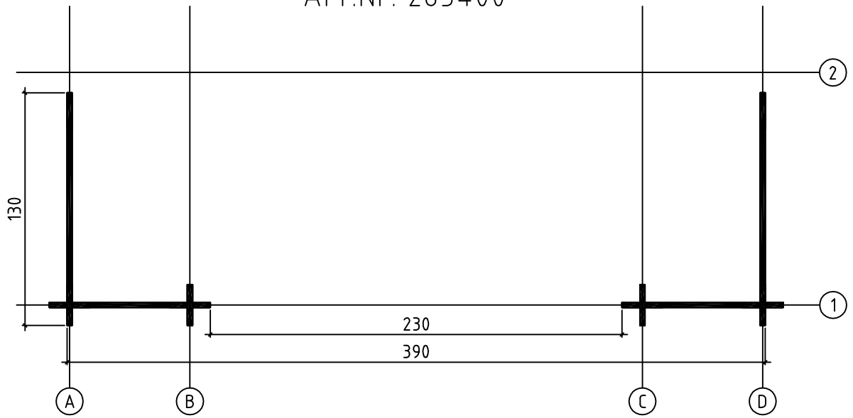
GROUNDPLAN - GRUNDPLAN - PLAN DE MASSE
