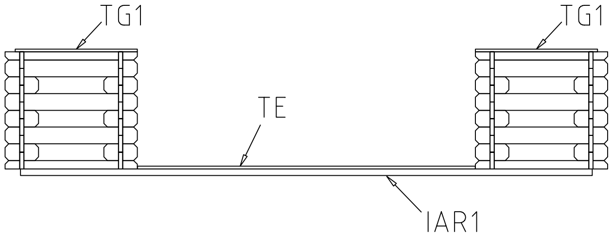
Side view - Seitenansicht - Élévation principale
